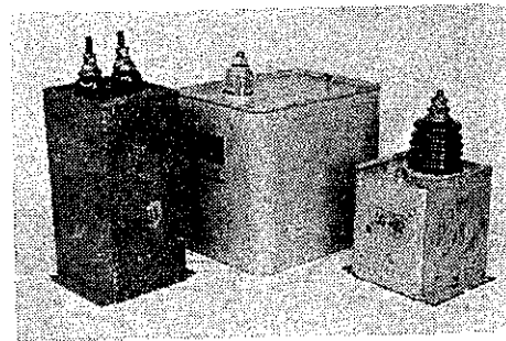
オイルコンデンサー (値段は荷造送共) 4 \mu F 4000V ¥ 700 1.5 \mu F 6000V ¥ 1,500 0.7 \mu F 7000V ¥ 300
