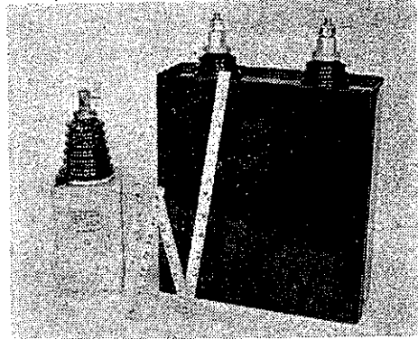
高圧オイルコンデンサー (写真左) 0.00025 25kV ¥ 500 (荷造送共)
