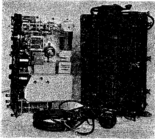
移動用送受信機 2~8 Mc バッテリーケース、レシーバー、電鍵、アンテナ、スペアパーツ共 程度上 ¥ 8,500 (荷造送共)
