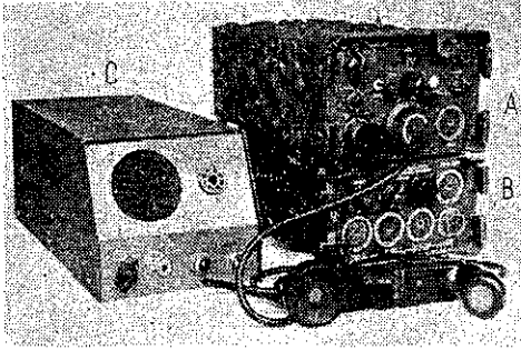
＜RT-70送受信機＞
